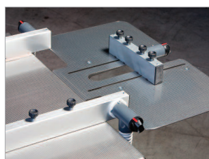
Plateau d'extension de la table d'alimentation pour formats longs.
